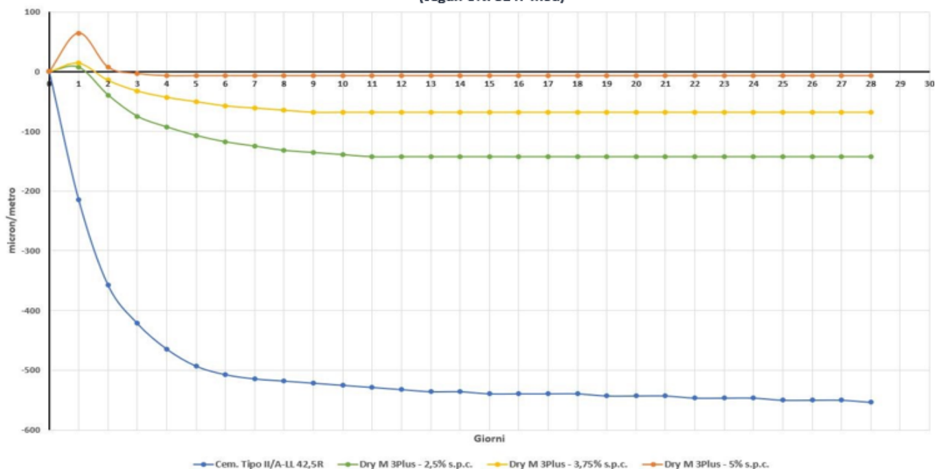
Dry M 3Plus -EXPANSIÓN/RETRACCIÓN LIBRE DEL MORTERO (según UNI 8147 mod)
