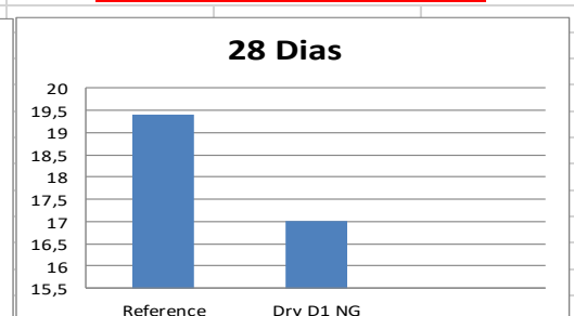
Desgaste/abrasão da superfície (mm)
