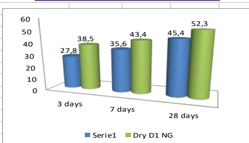
Resistência F ck por compressão -(Mpa)
