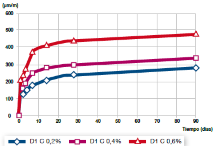
HORMIGONES CON D1 C EXPANSIÓN CONTRASTADA (SEGÚN UNI 8148)
